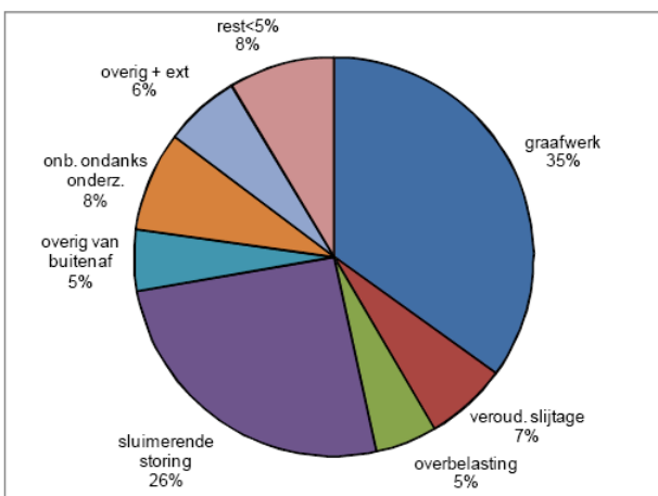
Storingsoorzaken laagspanning, 2008
